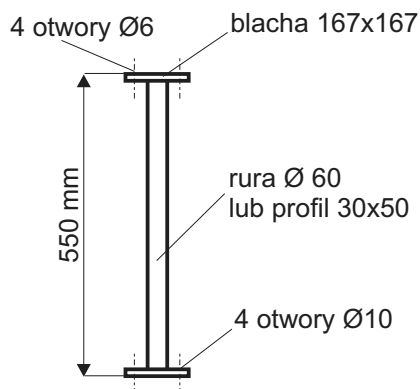
ilość podpór do montażu - 2 szt.
