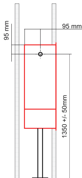
w ścianach z płyt kartonowo-gipsowych oraz jako wolnostojący z zastosowaniem podpór
